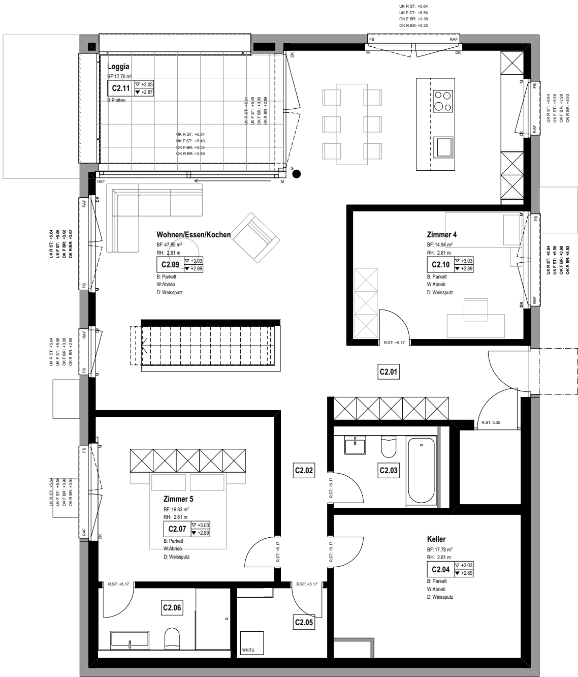
Grundriss Obergeschoss
