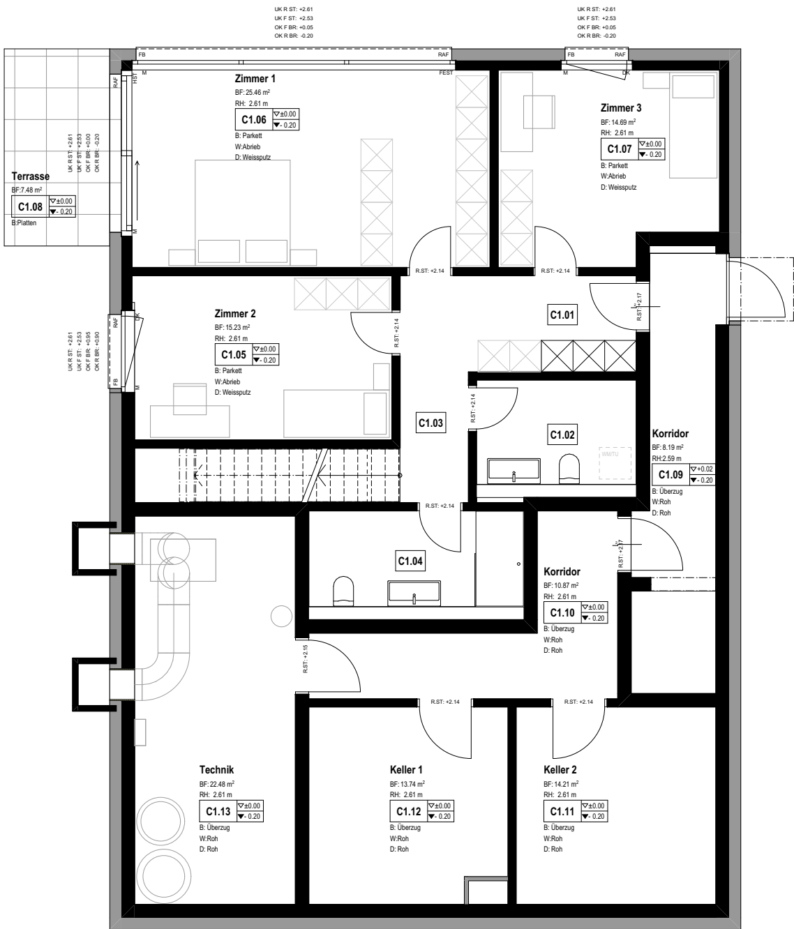
Grundriss Erdgeschoss
